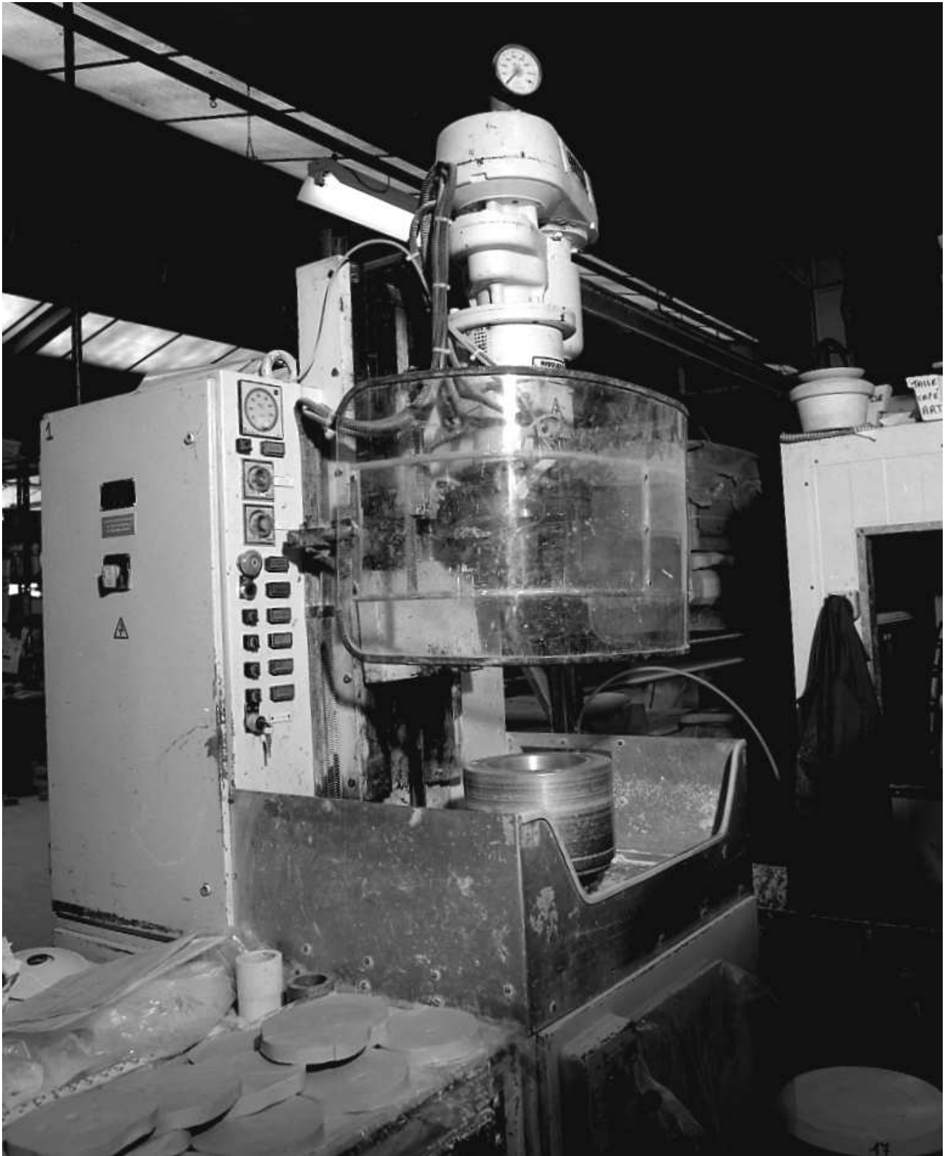
Fig.1 Vue de l'une des deux machines Roller du constructeur Dorst (machine n° 36121V).
